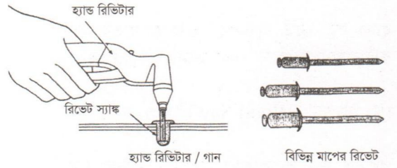
চিত্র ১.৩৪ : হ্যান্ড রিভিটার ও রিভেট
